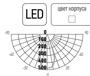
PSP-S 7W
