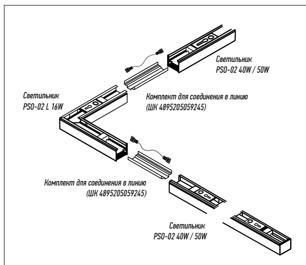
Схема соединения светильников PSO-02 с помощью светильника PSO-02 L
