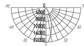
PTR 0130-2 30W
