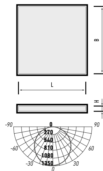
PPL SPEC1 OP 36W
