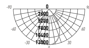
PHB 03 PRO-5 150W
