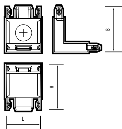
MTR16 CV-BL Коннектор черный V-обр.
