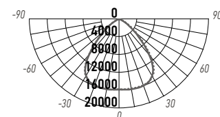
PHB 06 PRO-5 200W 90°
