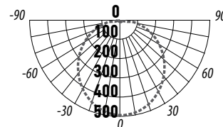
PBH PC LV 18W
