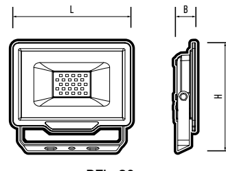
PFL-C3
