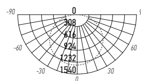
РР0-03 1200 40W
