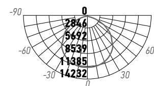
PFL-V 300W
