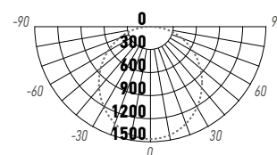
PPL PRO-5 595/R OPAL 30W
