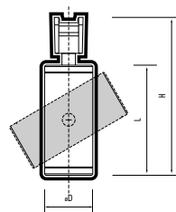
MTR16 2320A
