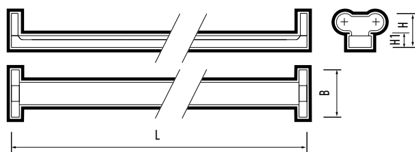
РР0-Т8 2Х1200
