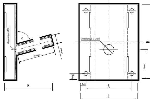
КРОНШТЕЙН НА СТОЛБ для PSL D40*1.5 ПОД БАНДАЖНУЮ ЛЕНТУ
