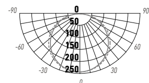
PPL-S 15W
