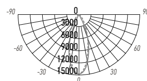
PTR 0325 25W
