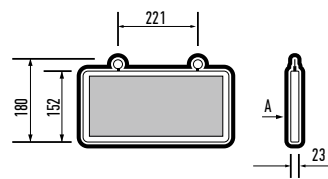
PEL 103-1 3W 1.2V IP20 ОДНОСТОРОННИЙ БЕЗ НАКЛЕЙКИ
