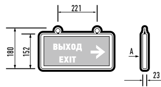
PEL 102-2 3W 1.2V IP20 "ВЫХОД-EXIT" / СТРЕЛКА НАПРАВЛЕНИЯ
