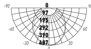
PTR 4620 20W
