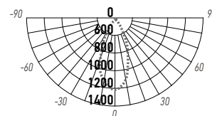
MTR16 1412 12W
