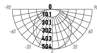
PTR 4520 20W
