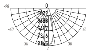
PTR 0728 28W 15°
