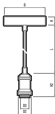
RETRO патрон PLC 01
