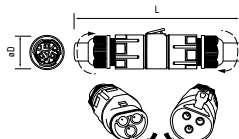
PCC-I3-FD 3x1.5 16A IP68
