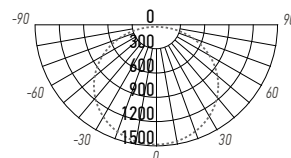
PWP-C3-E1 36W
