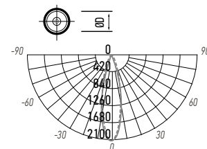
PTR 2310 10W
