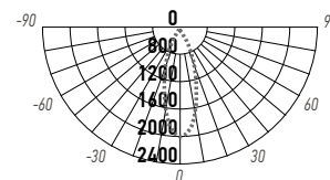
MTR16 1212 12W
