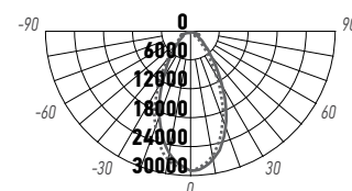
PHB 06 PRO-5 200W 60°
